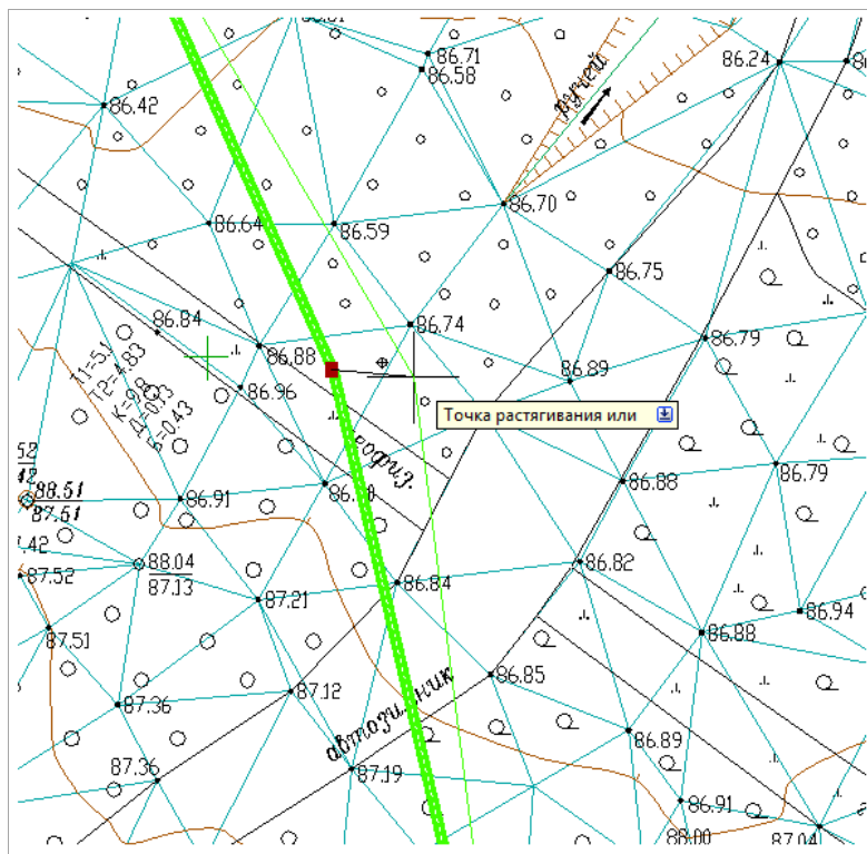
Рис. 23. Для быстрого и удобного редактирования геометрии объект Трасса содержит «ручки редактирования».
