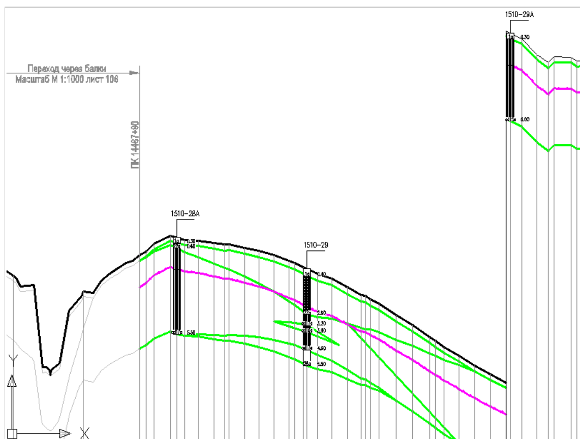
Рис. 56. Если геологическая линия проходит через сброс, то в местах сбросов на изображении геологии размещаются разрывы. При этом в модели данных геолиния и сам объект остаются целостными.
