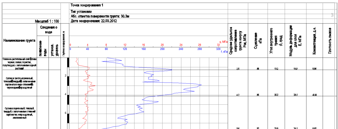
Рис. 85. Примеры литологических разрезов (геологических колонок).
